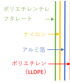
(PET/NY/AL/LL)
