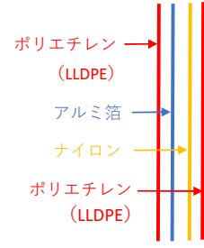
(LL/AL/NY/LL)
