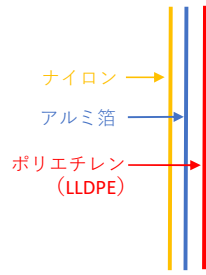
(NY/AL/LL)
